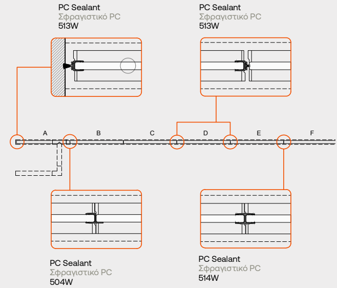
Horizontal sealing sections with sash joint detail Οριζόντια τομή με λεπτομέρειες σφράγισης
