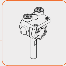
S.S. roller carrier with S.S bearings Βαγόνι ανοξείδωτο με ράουλα και ανοξείδωτα ρουλεμάν 729.110.11
