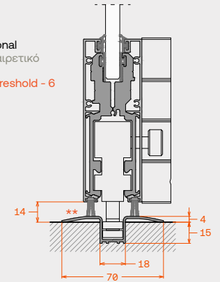
Vertical Section / Κάθετη Τομή
