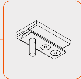
S.S. upper pivot Ανοξείδωτο άνω μύλι 529.226.11
