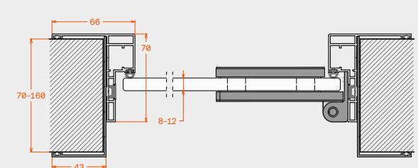
Horizontal section Οριζόντια τομή
