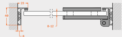
Horizontal section Οριζόντια τομή
