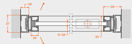
Horizontal section Οριζόντια τομή
