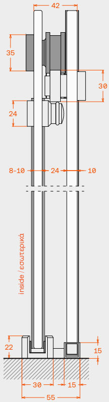
Vertical section Κάθετη τομή
